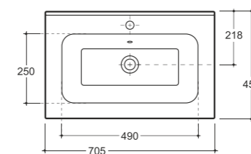
УМЫВАЛЬНИК ЖЕНЕВА 70 ВСТРАИВАЕМЫЙ WASH-BASIN GENEVA 70 PLUGGABLE
