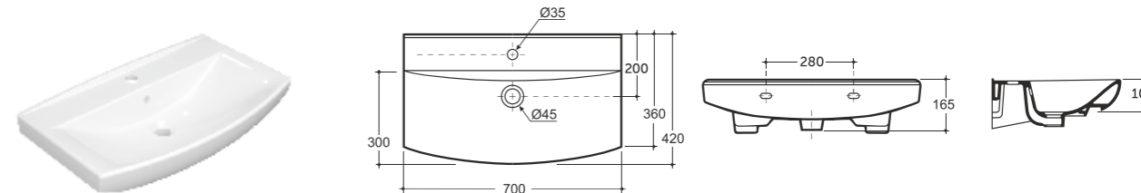
УМЫВАЛЬНИК МЕБЕЛЬНЫЙ КЛЕРМОНТ 70 SEMI-RECESSED WASH-BASIN CLAREMONT 70
